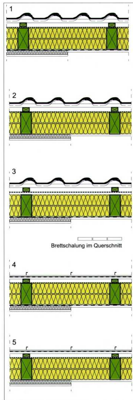
Bild 6.2 Konstruktionsprinzipien nach DIN 68 800-2 für Dächer der Gefährdungskategorie GK 0. Weitere Erläuterungen siehe untenstehende Legende.
