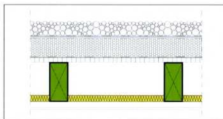
Bild 9.2 Flachdach GK 0 nach DIN 68 800-2 mit raumseitiger Bekleidung: Wärmeschutz überwiegend oberhalb der Decke angeordnet (Dämmmaterial beliebig), keine dampfsperrenden Schichten innerhalb des eigentlichen Deckenquerschnitts, an der Deckenunterseite möglichst diffusionsoffene Bekleidung (Gipsplatten, Brettschalung), evtl. zusätzliche Dämmschicht im Gefach aus mineralischen Faserdämmstoffen nach DIN 18 165-1 oder von Dämmstoffen mit Verwendbarkeitsnachweis
