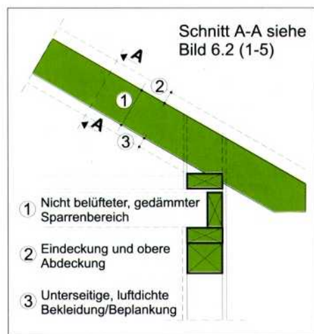
Bild 6.1 Überblick über die einzuhaltenden konstruktiven Bedingungen nach DIN 68 800-2 für Dächer der Gefährdungskategorie GK 0
